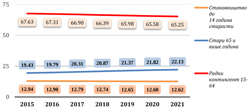
Проценат становништва општине Бачка Топола 2015.-2021. година- по старосним групама
